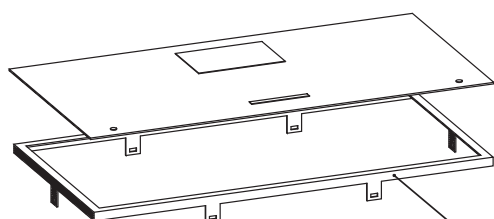
Kabeleinführungsplatte Typ Ic
